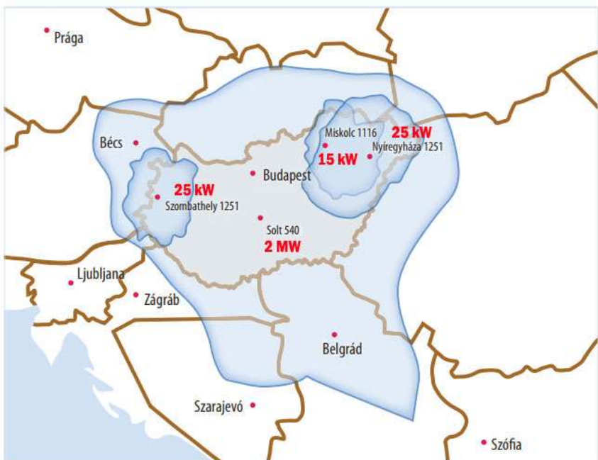
mr1-Kossuth lefedettségi térképe (adatok kHz-ben) Nappali lakossági ellátottság: 100%
