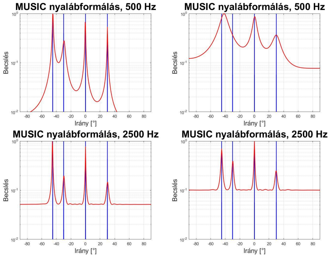
9. ábra: MUSIC nyálábformálás zajmentes (bal) és 20 dB jel-zaj viszonyú (jobb) esetben, 500 Hz (fent) és 2500 Hz (lent) vizsgálati frekvencián.
