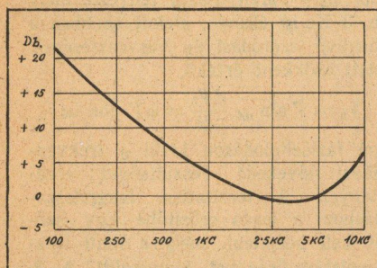
④ Mágneses hangleadó erősítő karakterisztikája.
