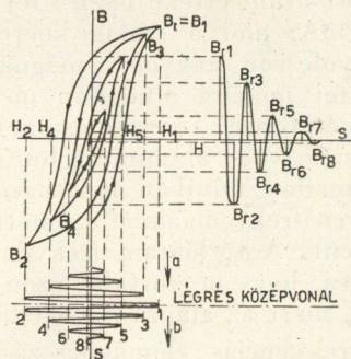
7. ábra. A nagyfrekvenciás törlés folyamata a a légréshöz közeledve b a légréstől távolodva B_{r1}, B_{r2} a szalag egy pontjának remanenciája az út függvényében
