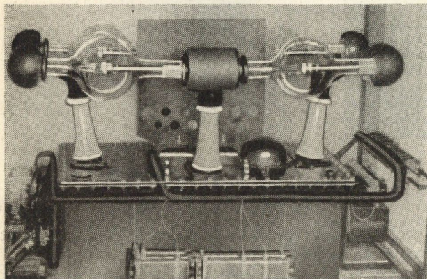
9. ábra 115 kV-os röntgentranszformátor ráépített négy szelepesővel Grätz-kapcsolásban 500 mA pillanatnyi terhelésre
