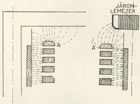
13/b ábra Erőtér gömbölyített szélű tekercsvégeknél és legömbölyített élű járómmal
