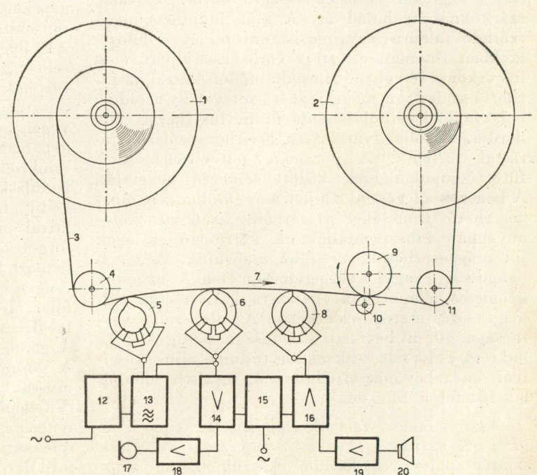
1. ábra. A mágneses hangrögzítő berendezés elvi felépítése
