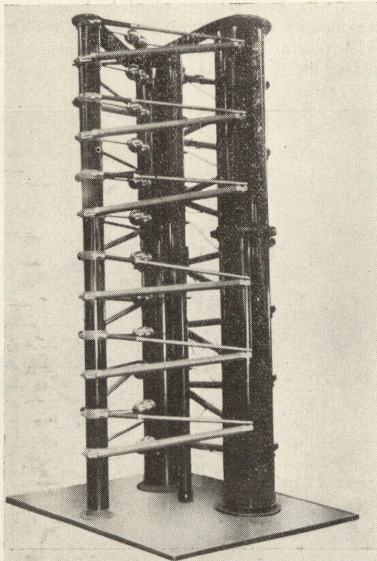
6. ábra 1500 kV-os lökésgeneresztő. Häfel-gyártmány
