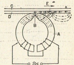
2. ábra. Mágneses felvevőfej A permalloy félgűrű B nem mágnesező betét C alapszalag (mérétei erősen nagyítva) D mágneses bevonat E a szalag mozgási iránya
