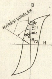
6. ábra. A remanencia csökkenése a zárt mágneses tér nyitásával \alpha_1, B_{r1} kis légrés esetén \alpha_2, B_{r2} nagy légrés esetén
