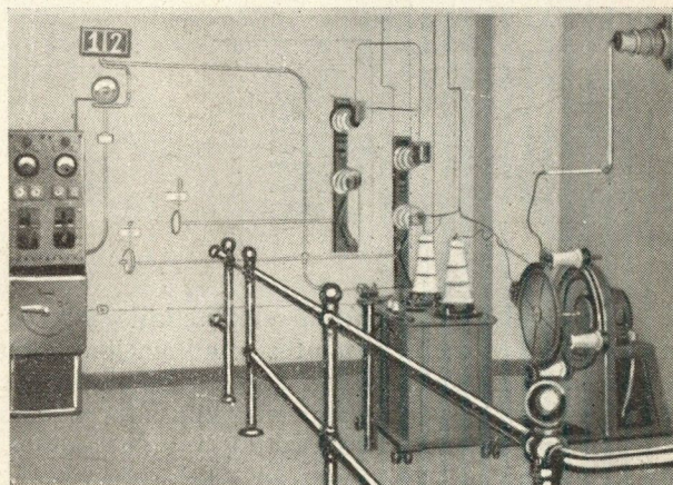
11/a ábra Villamos szűrő táplálására épült forgó egyenirányító: a anforrás
