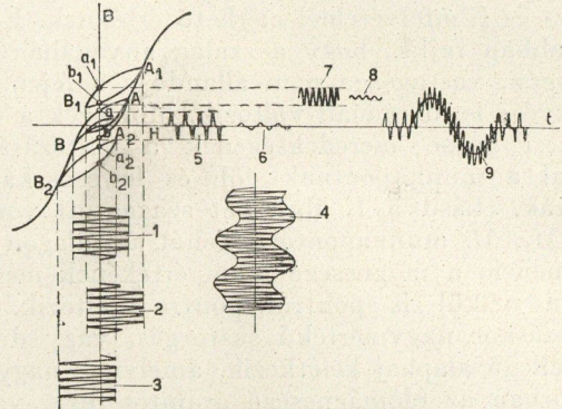
8. ábra. Nagyfrekvenciás előmágnesezés
