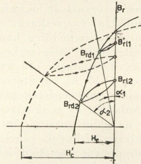
12. ábra. A szalag demagnetizálódása
