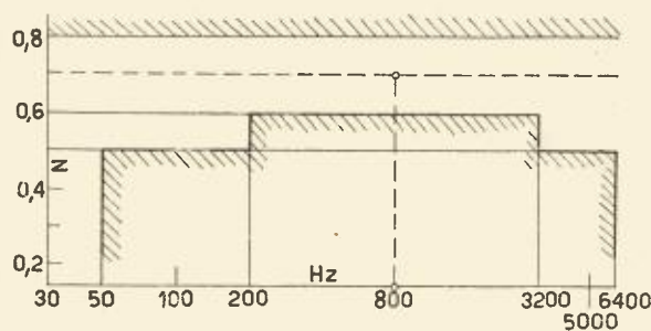
2. ábra. CCIF ajánlás »régípusú« zeneközlítő áramkörök szinttűréseire határ-erősítőállomás kimenetén
