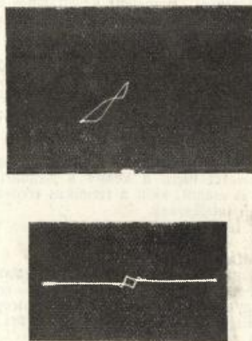
16. ábra. Sértetlen és meghajlított permalloy C lemez differenciagörbéje. A rugalmasság határán túl igénybevett anyag kezdeti permeabilitása és telítési indukciója csökken.
