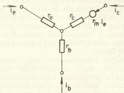
4. ábra. Tranzisztor csillaghelyettesítő képe.
