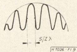
9. ábra. Interferométer-antenna iránykarakterisztikája
