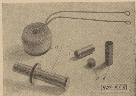
9. ábra. Magnéziumból folytatott fiolák a) szerszám alsórész; b) tüske; c), e) kész munkadarabok; d) előgyártmány
