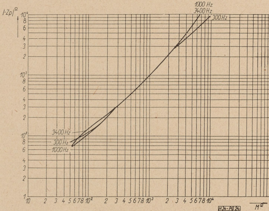
24. ábra. A valós vonalutánzzat transzformálása a vonalutánzzat értékeinek függvényében, párhuzamos jellegű negatív impedanciájú erősítő esetében
