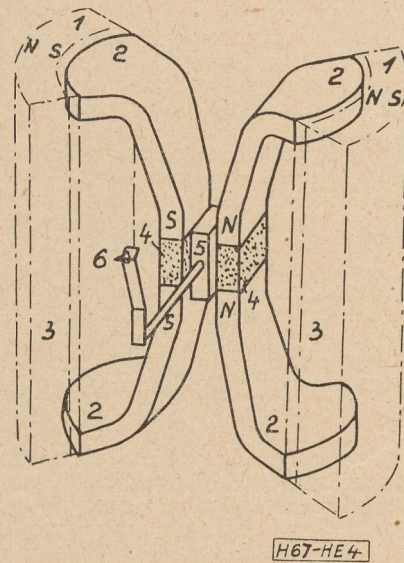
4. ábra. Antimágneses anyag
