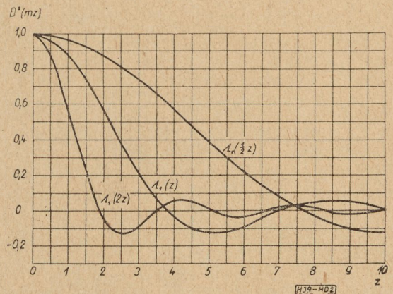
2. ábra. A D^*(z) = \Lambda_1(z) ; D^*(m_e z) = \Lambda_1(z) ; D^*(m_g z) = \Lambda_1\left(\frac{z}{2}\right) , természetes és módosított irányítási tényezők
