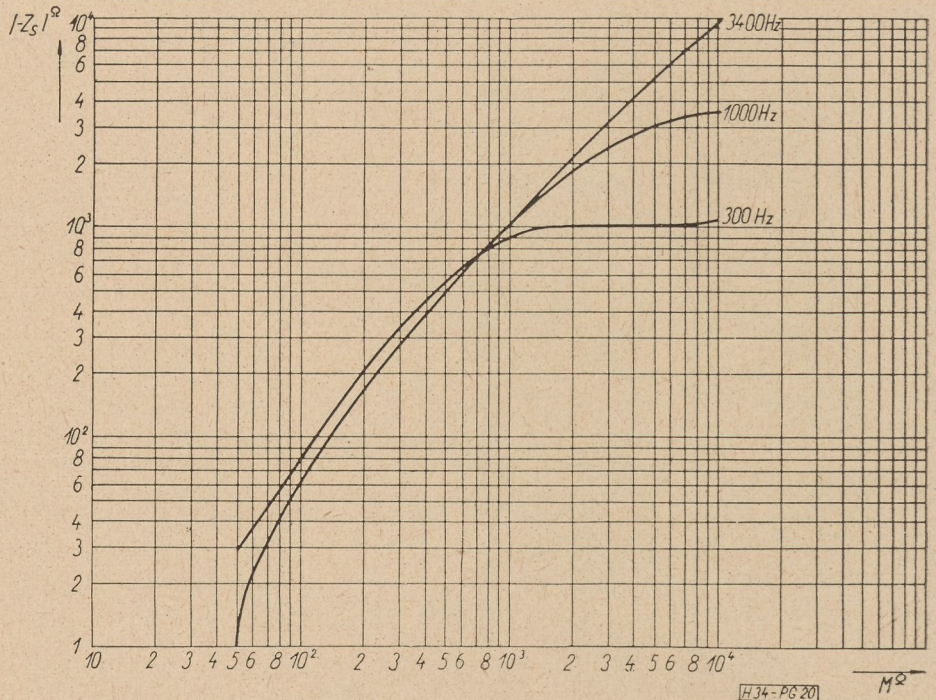
20. ábra. A valós vonalutáncat transzformálása a vonalutáncat értékek függvényében soros jellegű negatív impedanciájú erősítő esetében
