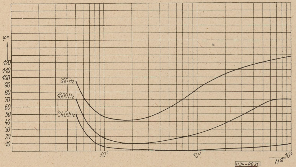
21. ábra. A valós vonalutáncat transzformálásának fázisszöge a vonalutáncat értékeinek függvényében, soros jellegű negatív impedanciájú erősítő esetében
