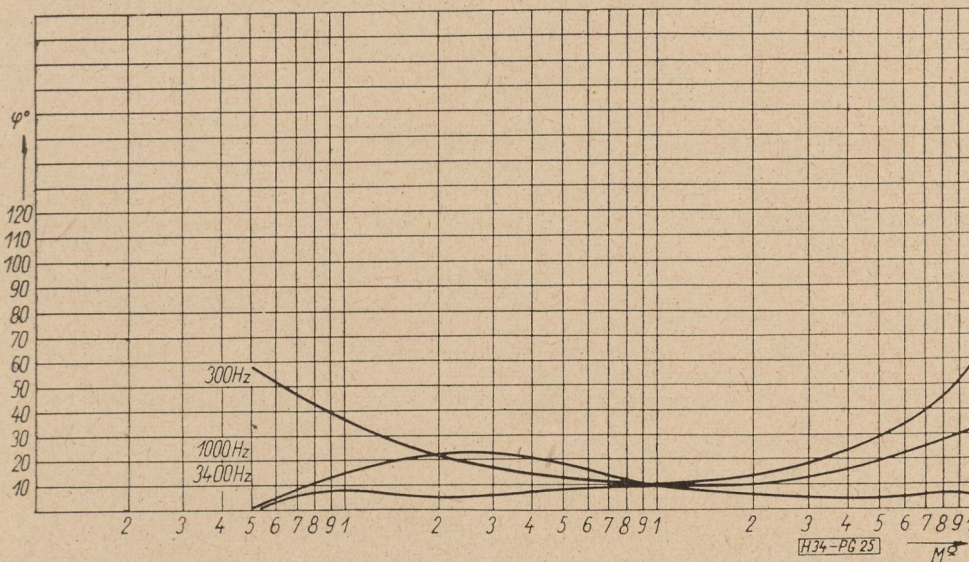
25. ábra. A valós vonalutánzzat transzformálásának fáziszöge a vonalutánzzat értékeinek függvényében, párhuzamos jellegű negatív impedanciájú erősítő esetében
