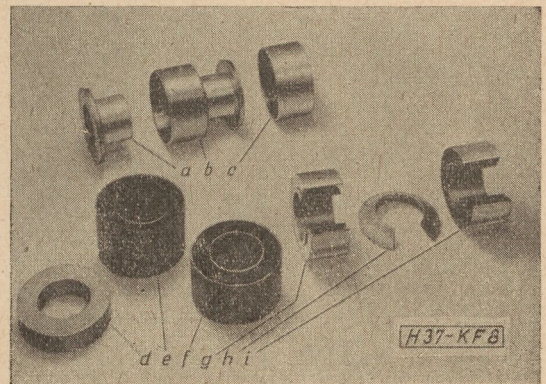
8. ábra. Vörösrézről hidegfolytatott „S” dugattyú a), b), c) tömör anyagból esztergált munkadarabok; d) előgyártmány; e) hidegfolytatott munkadarab; f) utánmunkált munkadarab; g), h), i) metszetek
