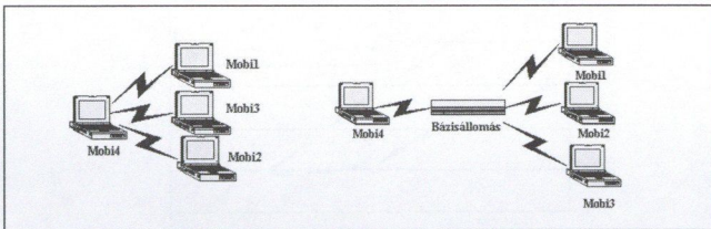
5. ábra Mérési elrendezés négy mobil állomással ad hoc és bázisállomás üzemmódban
