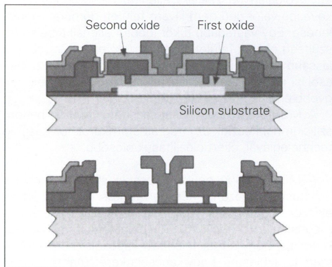
3. ábra Felső kép: maszkolással felvitt rétegek. Alsó kép: a maratás után visszamaradt bonyolult struktúra (forrás: [4]).
