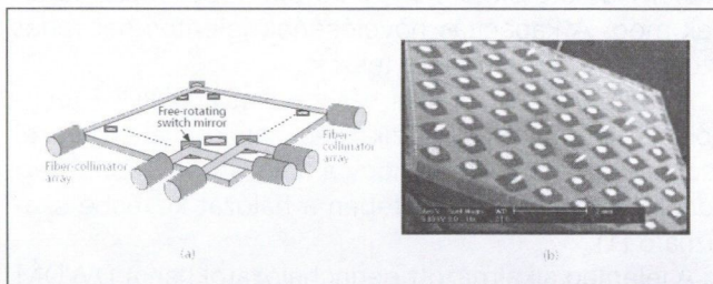
1. ábra a) 2D MEMS kapcsoló felépítésének tematikus rajza b) Egy AT&T 8x8-as MEMS kapcsoló (forrás: [3])
