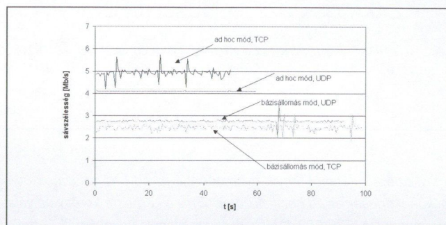
3. ábra Átviteli sávszélesség különböző üzemmódokban
