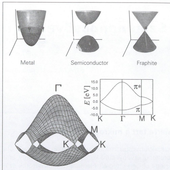
2. b. ábra Balra a fém, félvezető és a fél fémes tulajdonságú grafit sáv szerkezetének sematikus rajza. Míg a jó vezető fém esetében a vegyértéksáv és a vezetési sáv állapotai átfednek és a Fermi szintig betöltöttek, a félvezetőben a két sávot egy tilos sáv választja el, ahol nincsenek megengedett elektronállapotok. Vezetési elektronok így csak gerjesztéssel keletkezhetnek.
