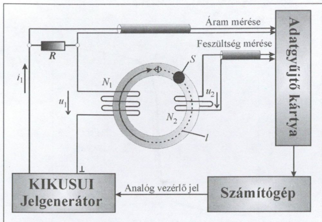
1. ábra A mérési elrendezés
