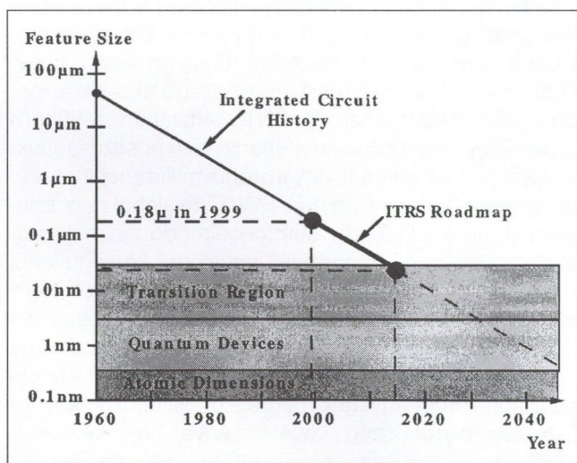
1. ábra A kritikus struktúra-méretetek csökkenése az integrált áramkörti technológiában a Moore-törvény érvényesülése következtében. Az előrejelzések szerint századunk második évtizedében a Si technológia fejlődése az ún. átmeneti tartományban kritikus szintre érkezik.
