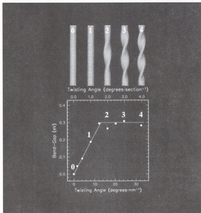
6. ábra A tilos-sáv szélességének változása a nanocső csavarodása következtében. Az abszcisszán a csavarási szög látható a fok/nm egységben.
