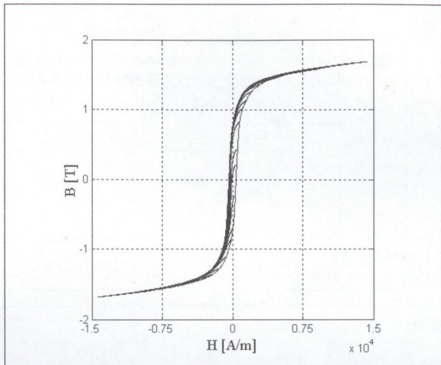
3. ábra A mért elsőrendű visszatérő hiszterézis görbék
