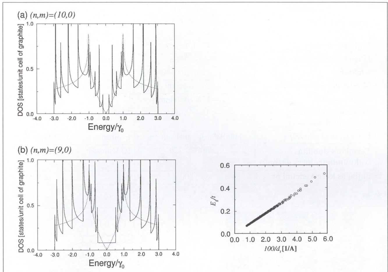
5. ábra A fémes (10,0) (a) és a félvezető (9,0) cikk-cakk nanocső állapotsűrűség-eloszlása (ld. tilos sáv!) (b) a jellemző egydimenziós szingularitásokkal (M. Dresselhaus elméleti számításai alapján). Pontvonallal a kétdimenziós grafit állapotsűrűség-eloszlása látható. Jobbra a nanocsőekben a tilos-sáv szélesség átmérő-függését ábrázolták ugyancsak elméleti számítások alapján.
