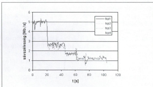
14. ábra 4 TCP adatfolyam késleltetve sávszélessége
