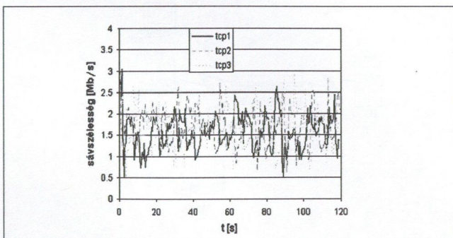
6. ábra Ad hoc üzemmódban 3 TCP adatfolyam sávszélessége
