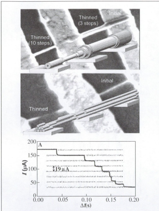
11. ábra Az IBM kutatói által kidolgozott ún. „konstruktív destrukció” módszerének ábrázolása egyfálú félvezető nanocsövek kiválasztására sokfálú MWNT nanocsövekből (fent) és egyfálú SWNT nanocső-kötegekből (lent). Az oxidált szilíciumszelvényen fekvő sokfálú nanocsöveken és egyfálú nanocső-kötegeken keresztül arany fémkontaktusokat alakítanak ki. A félvezető nanocsövek kikapcsolása után adott feszültségről áramot kényszerítenek a fémes CNT-ken keresztül, ami ezek fokozatos letörését, ill. megszakítását eredményezi. Az alsó görbén jól követhető az áram időfüggő alakulása egy-egy héj eltávolítása után. A felső képen az eljárás vázlata mellett a SEM képen jól látható a végeredmény is.
