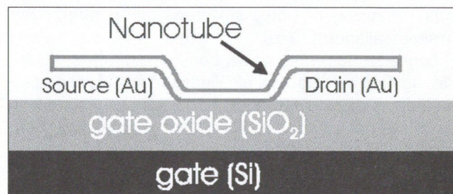
8. ábra Térvezérelt szerkezetek egyfalú félvezető nanocsövekből (CNTFET) oxidált szilíciumszeleten arany source-drain kontaktussal. A CNTFET gate-elektrodja maga a Si szubsztrát [2].
