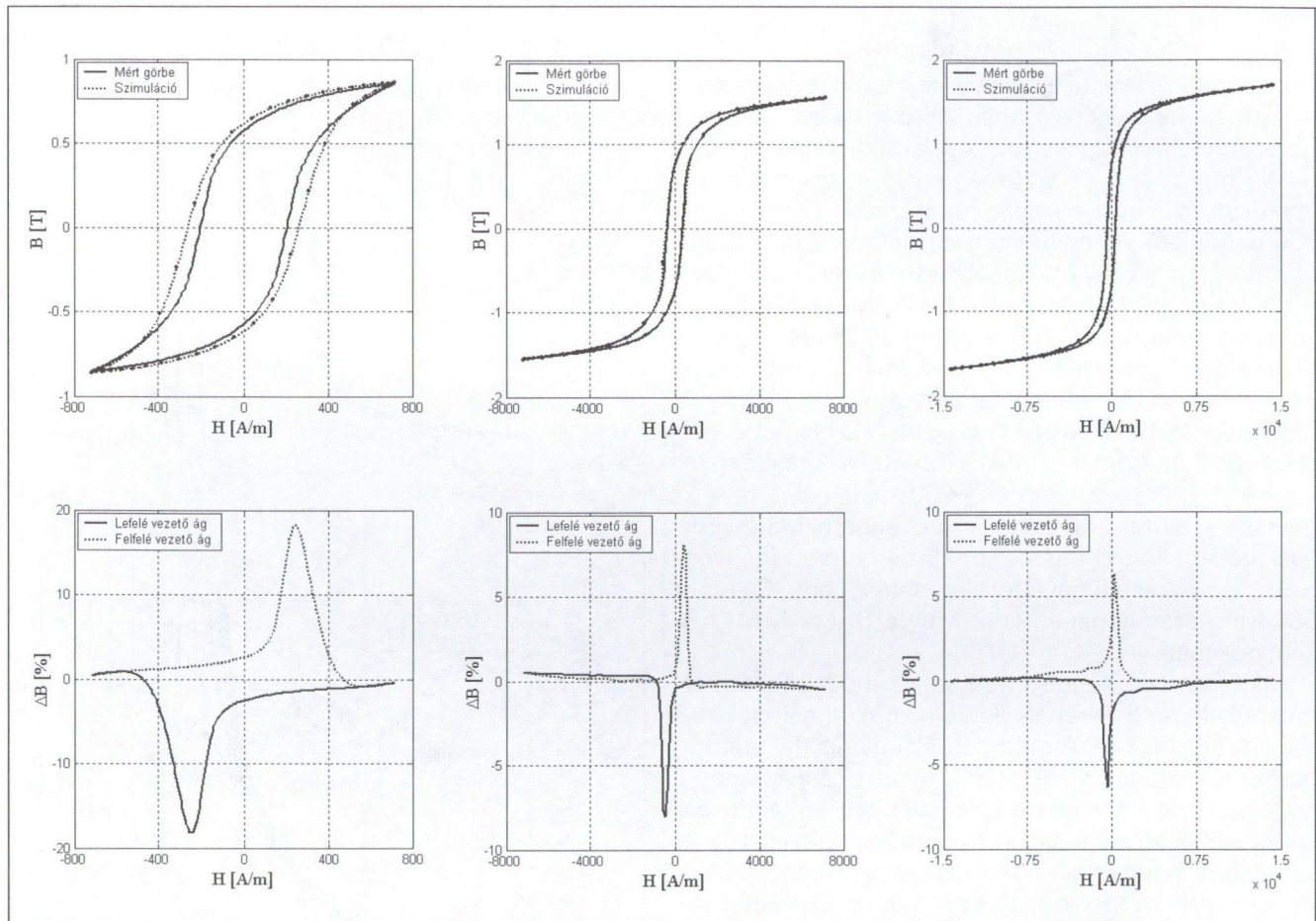
6. ábra A mért koncentrikus hiszterézis görbék és a szimuláció eredményének összehasonlítása
