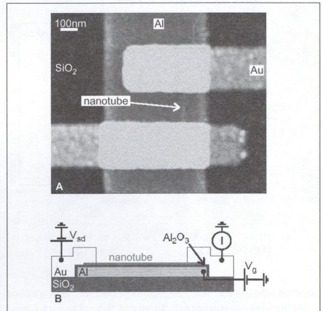
12. ábra CNTFET szerkezet kialakítása oxidált szilíciumon futtatott Al vezetéken a rája képződő alumíniumoxidot használva gate elektródaszerkezetként arany kontaktusok között. Fent a szerkezet nagyfelbontású pásztázó elektronmikroszkópos képe, lent a térvázelt eszköz vázlata. A be- és kikapcsolt állapot között >100.000-szeres ellenállásarányt kaptak [3].
