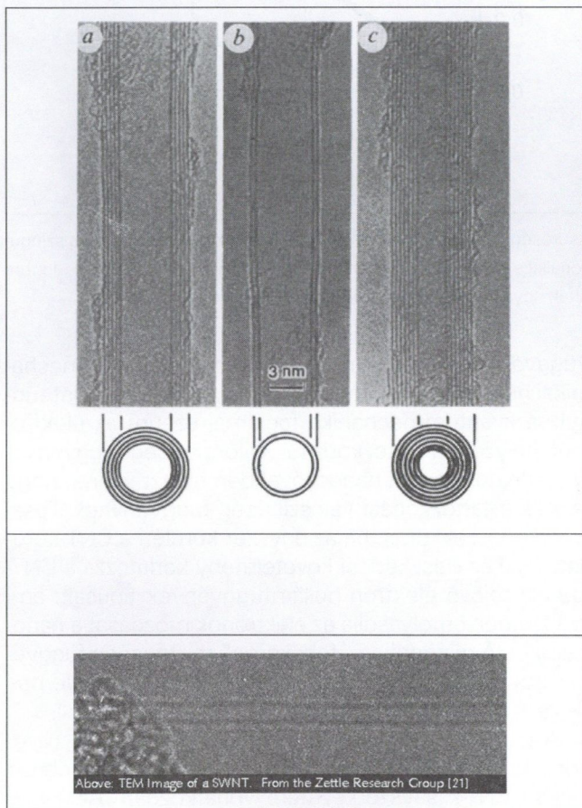
3. ábra Felül az első, 1991-ben publikált transzmissziós elektronmikroszkóp felvételek sokfalú szén (MWNT) nanocsövekről az Iijima-csoportban [5]. Az alsó felvételen egy egyfalú (SWNT) nanocső elektronmikroszkópos képe látható.
