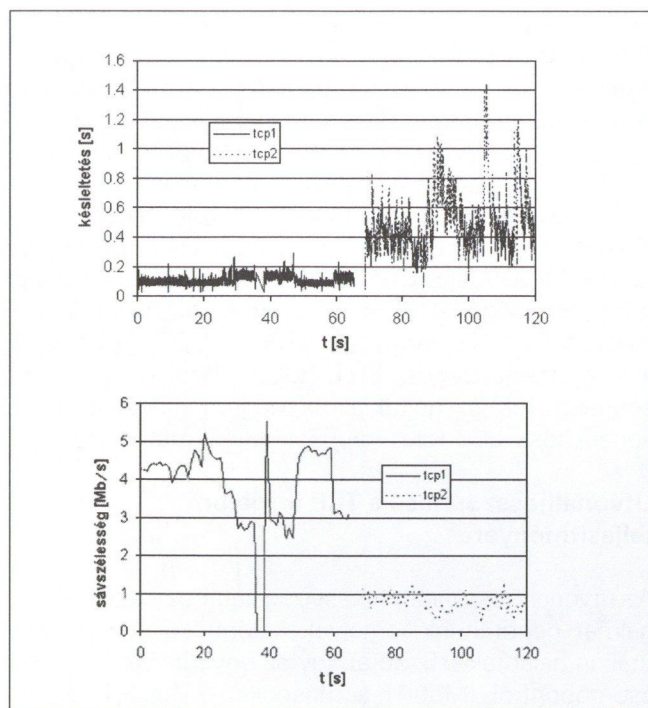
16. ábra Késleltetés és sávszélesség két TCP folyamattal
