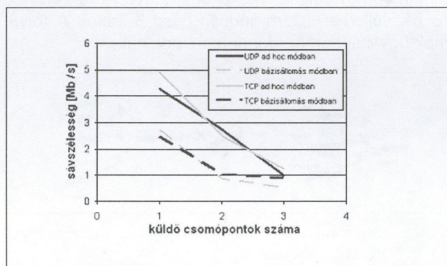
11. ábra Sávszélességek változása az adó csomópontok számának függvényében: TCP, UDP (AH –Ad Hoc mód, AP – Bázisállomás-mód)
