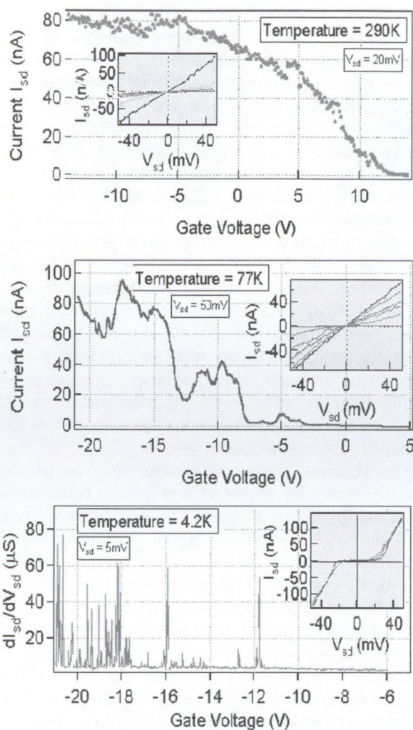
10. ábra A CNTFET bemenő-karakterisztikája és az ábrába ültetett kimenő jelleggörbéje három hőmérsékleten [2]. T=290\text{K} esetén, azaz szobahőmérsékleten a CNTFET viselkedése egyértelműen tranzisztor jellegű. T=4,2\text{K} , azaz hélium hőmérsékleten a jelleggörbe az egyelektronos tranzisztor (SET) működést mutatja. A T=77\text{K} nitrogén hőmérsékleten kapott eredmény átmeneti állapotnak felel meg [2].
