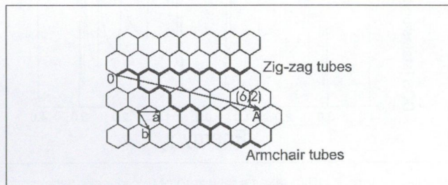
4. ábra A szén nanocsövek kiralitását vagy helicitását szemléltető ábra. A cikk-cakk tengelyre merőlegesen az ún. cikk-cakk nanocsöveket, a „karosszék” tengelyre merőlegesen össztekert grafitsíkból a karosszék-típusú nanocsöveket kapjuk. A két speciális esetben kívül a kiralitási vektor értékével jellemezhető a nanocső.
