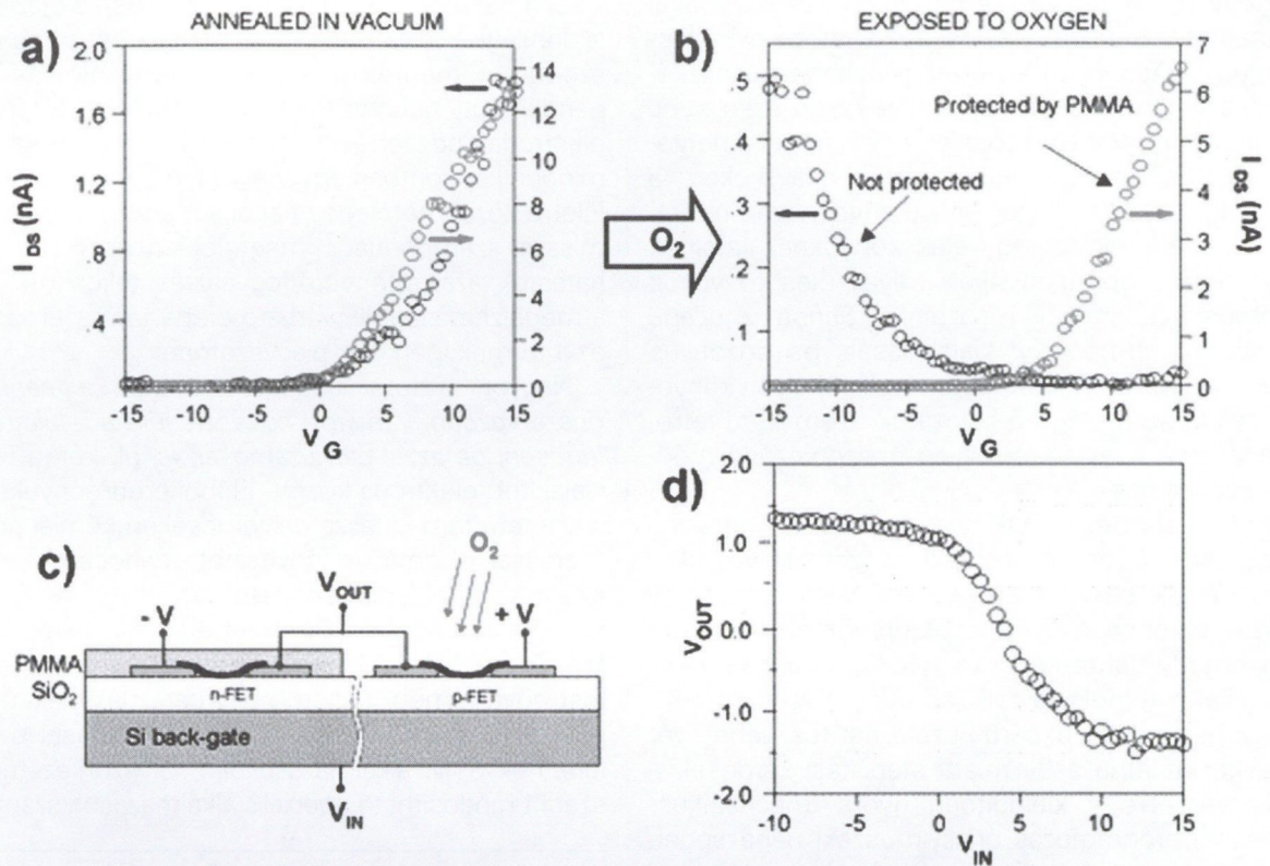
14. ábra Az IBM csoport eljárása komplementer CNTFET-ek megvalósítására d_t=1,4\text{nm} átmérőjű egyfalú SWCNT félvezető nanocsöveken, melyek sávzélessége E_g=0,6\text{eV} . Az (a) ábra I_{DS}=f(V_G) karakterisztikái mutatják az eredetileg p-csatornás CNTFET átalakulását rövid 400^\circ\text{C} -os vákuum-hőkezelés után. A folyamat a (b) ábra szerint oxigénben megfordítható (lyukvezetés), kivéve a PMMA réteggel védett eszközt. A (c) ábra egy p- és n-csatornás eszköz felhasználásával felépített intramolekuláris komplementer invertert mutat, melynek kimenő karakterisztikája a (d) ábrán látható [2].
