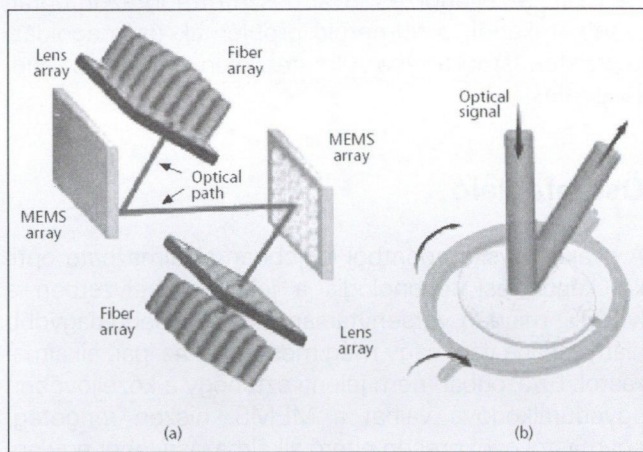
2. ábra a) A 3D MEMS kapcsoló felépítése b) A fény irányítása kardángyűrű segítségével (forrás: [3]).
