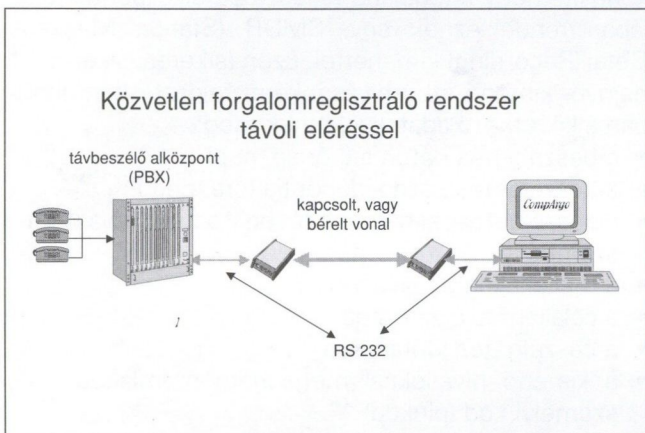
2. ábra Közvetlen forgalomregisztráló rendszer, távoli eléréssel
