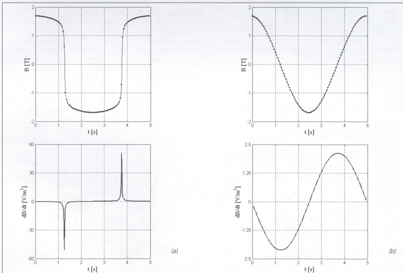
2. ábra A mérési pontok eloszlása és a mágneses indukció változásának alakulása (a) a direkt karakterisztika és (b) az inverz karakterisztika szimulációja alapján
