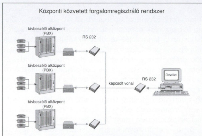
4. ábra Központi közvetett forgalomregisztráló rendszer helyi pufferrel
