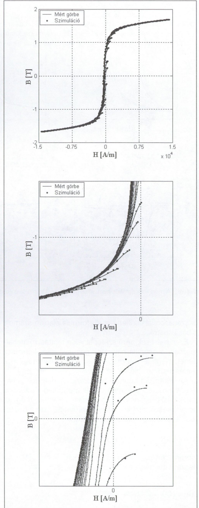
5. ábra A mért elsőrendű visszatérő görbék összehasonlítása a szimulációs eredményekkel
