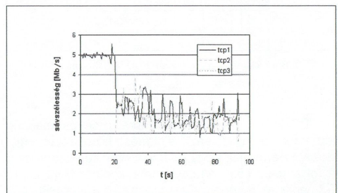
8. ábra Ad hoc üzemmódban 3 TCP adatfolyam 20 másodperces késleltetéssel
