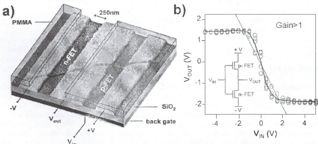
15. ábra Az IBM intramolekuláris komplementer CNTFET inverter képén (a ábra) oxidált Si szeleten egyfalú nanocső-köteg AFM képe látható 3 arany vezetékre fektetve. A két sorbakapcsolt CNTFET közül a jobboldali PMMA réteg borítja az oxigén hőkezelés alatt. Az n-csatorna adalékolása miatt a p- és az n-CNTFET küszöbfeszültsége megegyezik. A (b) ábrán az inverter erősítése 1,6, azaz egy további inverter vagy gyűrűoszillátor meghajtására is képes [2].
