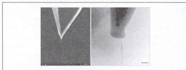
17. ábra Pásztázó mikroszondás tűk hegyén növesztett szén nanocsövek a pásztázó módszerek felbontásának javítására. Nem csak a laterális felbontást növelik meg, hanem mély barázdák alakhú letapogatását is lehetővé teszik [7].
