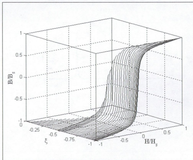
4. ábra Az elsőrendű visszatérő görbék előfeldolgozás után
