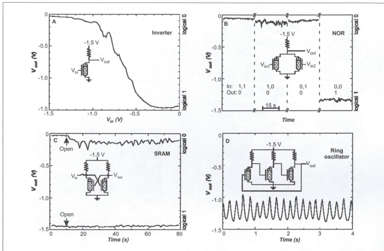
13. ábra CNTFET logikai kapcsolások külső terhelőellenállások felhasználásával. A logikai alapkiosztások, inverter, NOR kapu, sztatikus RAM cella, 3 fokozatú gyűrűs oszcillátor működése a megfelelő diagramokon követhető nyomon [3].
