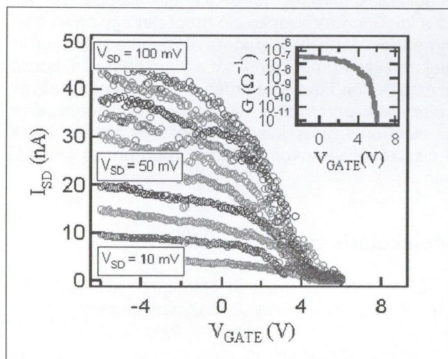
9. ábra A CNTFET bemenő karakterisztikái különböző V_{SD} előfeszítés mellett. A jelleggörbe alapján a normál állapotban nyitott csatornás, lyukvezetési működés egyértelműen megállapítható. A csatorna vezetőképességének változását a gate-feszültség hatására a beillesztett ábra mutatja.
