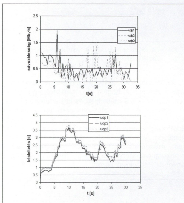
10. ábra Bázisállomás üzemmódban 3 UDP adatfolyam: sávszélesség, késleltetés
