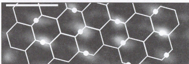
7. ábra Az egyfalú nanocsőben pásztázó alagútmikroszkópiával (STM) detektált hullámfüggvény térkép. A fehér vonalak a rávetített hexagonális atomrácsot szimbolizálják, a fehér pöttyök az elektronsűrűség maximum helyeinek jelzésére szolgálnak. Az elektron állóhullámok periodicitása eltér a rácsperiódustól [3].
