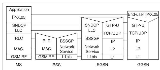
4. ábra A GPRS protokollkészlet felépítése
