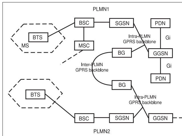
2. ábra A GPRS rendszer vázlatos felépítése
