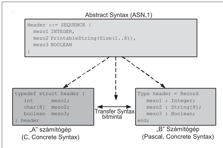
3. ábra A fenti példára vetített szintaxis hármas
