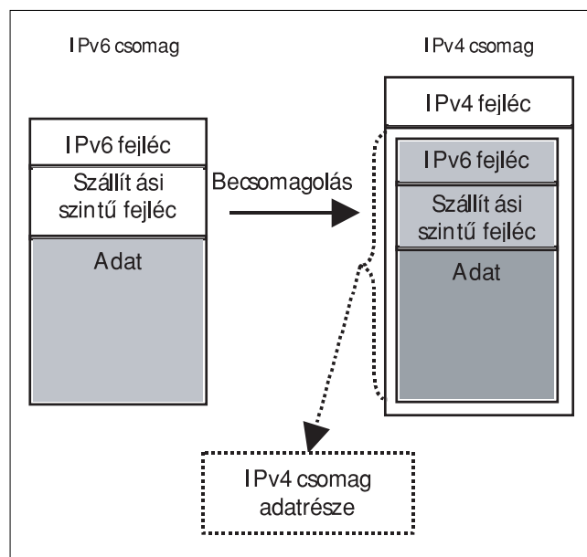
3. ábra IPv6-os protokoll IPv4-be ágyazása
