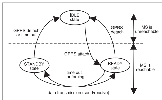
3. ábra Az MS állapotai, és azok kapcsolata
