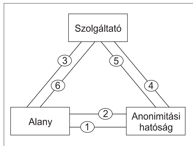
3. ábra Az anonim engedélyezés általános lefolyása az AH keretében
