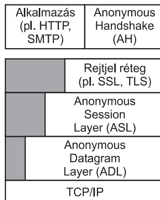
1. ábra Az általános célú biztonságos anonimitási architektúra rétegei
