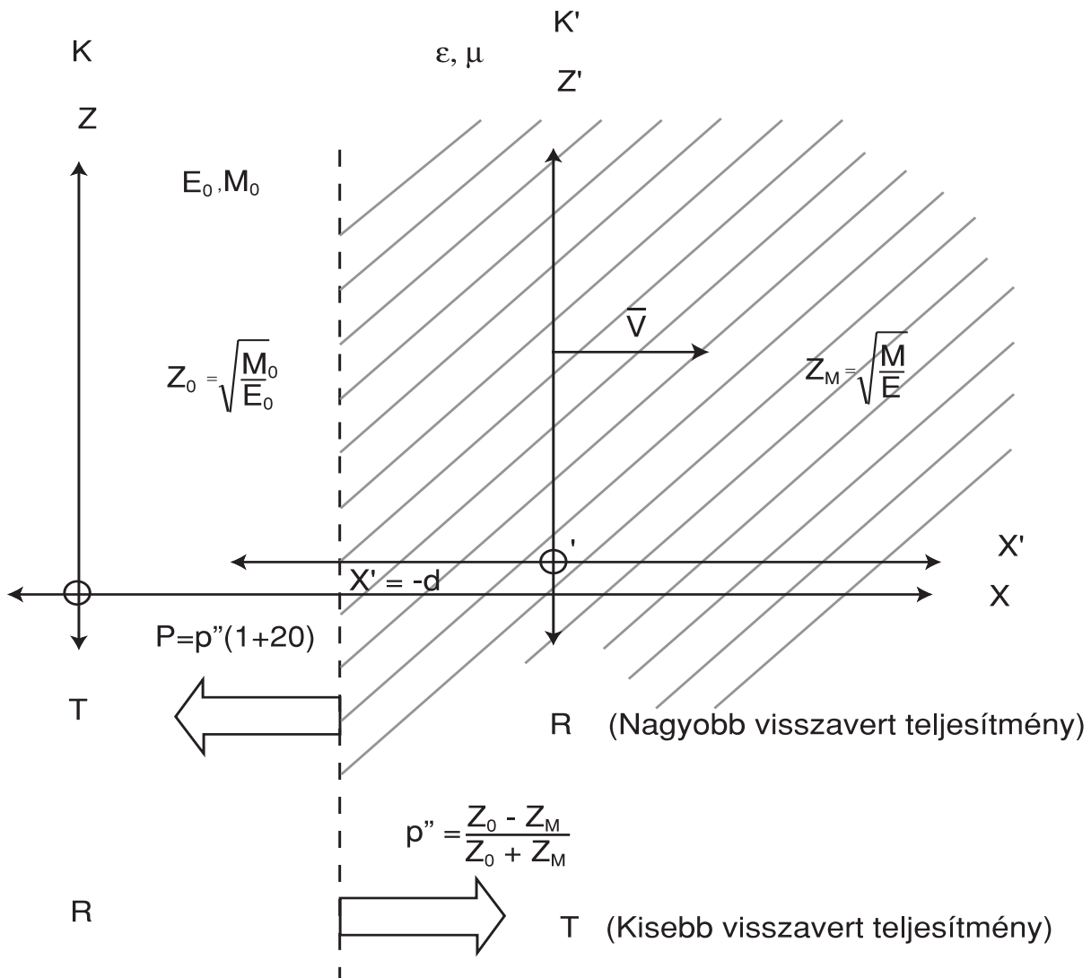
2. ábra Inhomogén tér
