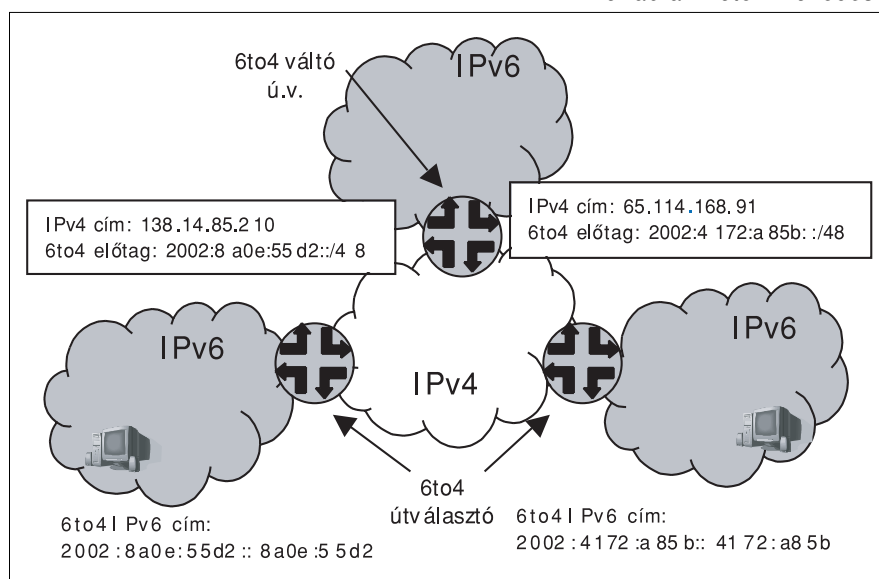
6. ábra A 6to4 működése
