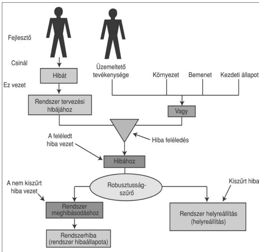
2. ábra A koncepcióbeli (vagy a tervezési) meghibásodásokra vonatkozó „hiba (tévedés)”, „hiba (hibaállapot)”, „hiba” és „meghibásodás” fogalmak közötti kapcsolat
