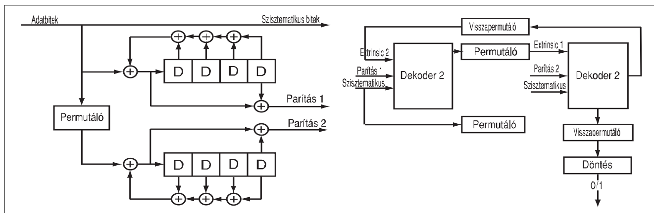
4. ábra Két konvolúciós kódolót tartalmazó Turbó-kódoló (balra) és dekódoló (jobbra)
