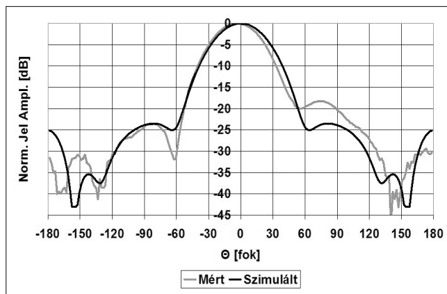
19. ábra H síkú dbiquad iránydiagramok
