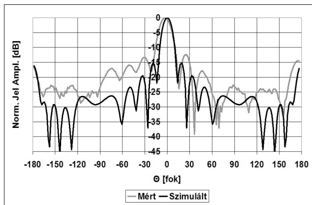
20. ábra H síkú quad6 iránydiagramok
