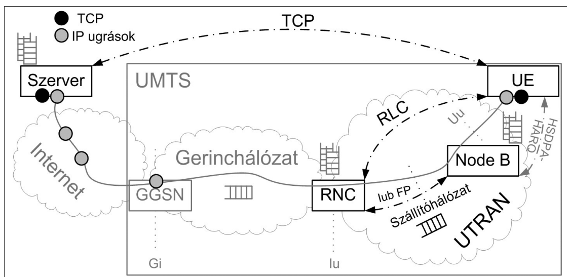
2. ábra Vezérlő hurkok a 3G/HSDPA-ban
